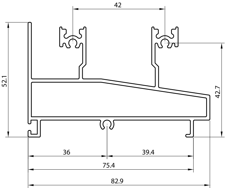
3402 RIEL INFERIOR CAMARA Peso : 1.465 Kg/M Espesor : 1.5 mm Largo : 7.25 Mt.
