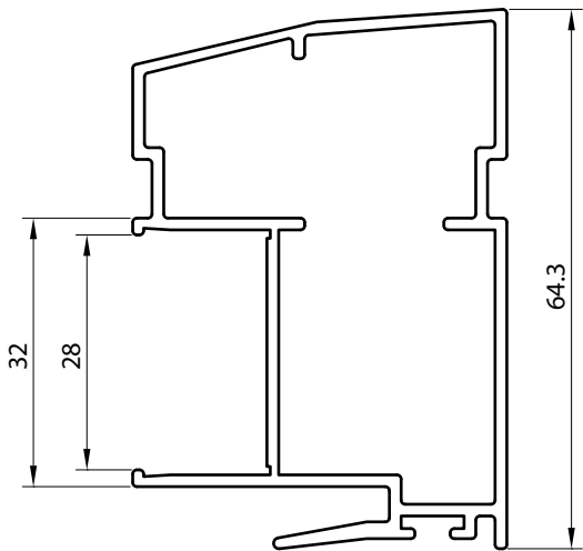
3408 TRASLAPO REFORZADO Peso : 0.981 Kg/M Espesor : 1.4 mm Largo : 7.25 Mt.
