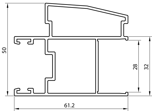
3406 PIERNA TERMOPANEL Peso : 1.061 Kg/M Espesor : 1.4 mm Largo : 7.25 Mt.
