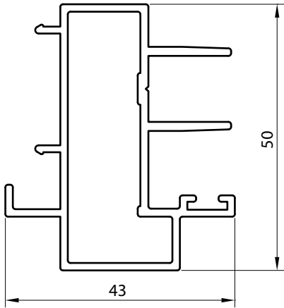
3411 CUARTA HOJA Peso : 0.838 Kg/M Espesor : 1.4 mm Largo : 7.25 Mt.
