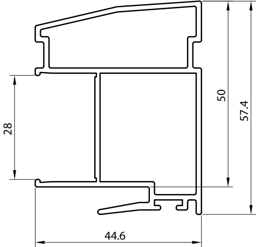
3407 TRASLAPO Peso : 0.982 Kg/M Espesor : 1.4 mm Largo : 7.25 Mt.
