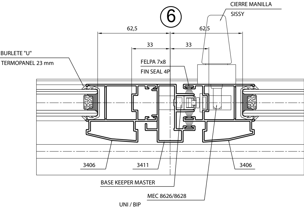
Corte Horizontal doble vidrio, encuentro a tope cuarta hoja.
