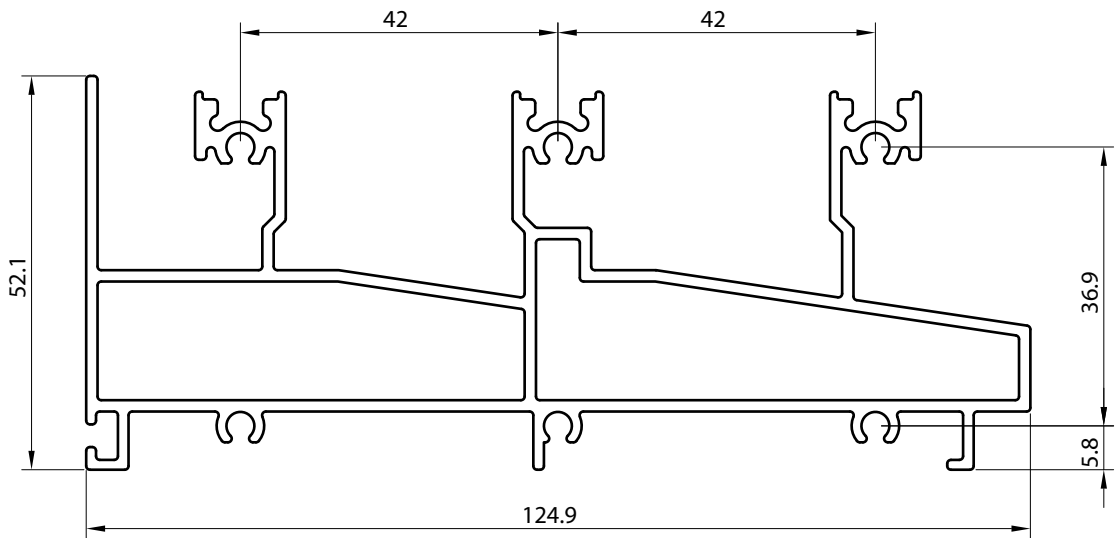
3412 RIEL INFERIOR 3 LINEAS Peso : 2.202 Kg/M Espesor : 1.5 mm Largo : 7.25 Mt.
