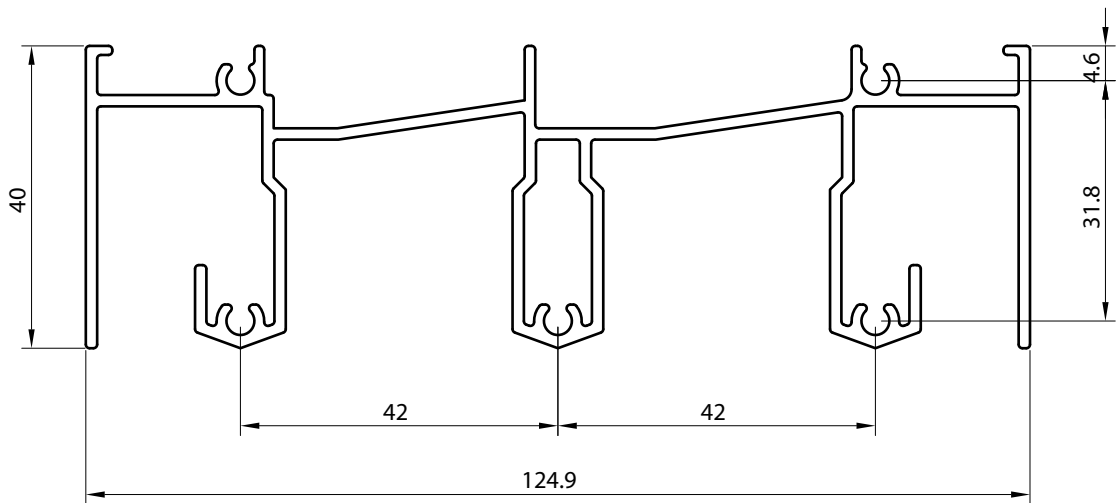
3413 RIEL SUPERIOR 3 LINEAS Peso : 1.692 Kg/M Espesor : 1.5 mm Largo : 7.25 Mt.
