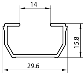
3409 ADAPTADOR MONOLITICO Peso : 0.217 Kg/M Espesor : 1.2 mm Largo : 6.05 Mt.
