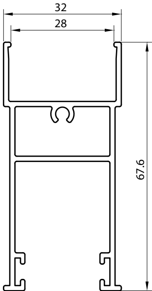
3405 ZOCALO REFORZADO Peso : 0.829 Kg/M Espesor : 1.4 mm Largo : 7.25 Mt.
