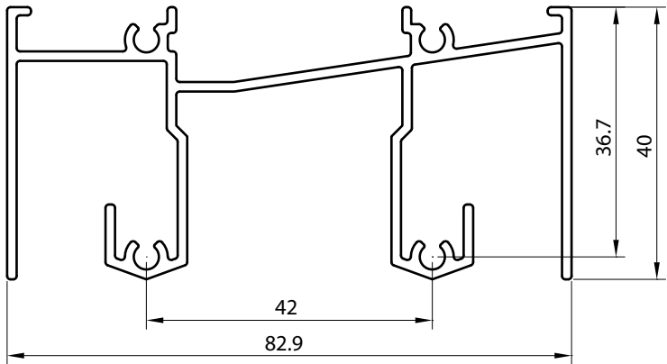
3401 RIEL SUPERIOR Peso : 1.133 Kg/M Espesor : 1.4 mm Largo : 7.25 Mt.
