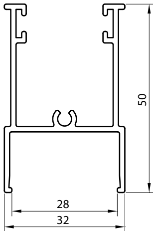
3404 CABEZAL Peso : 0.598 Kg/M Espesor : 1.4 mm Largo : 7.25 Mt.
