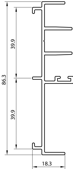
3403 JAMBA Peso : 0.732 Kg/M Espesor : 1.5 mm Largo : 7.25 Mt.
