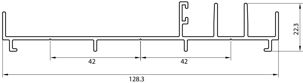
3414 JANMBA 3 LINEAS Peso : 0.922 Kg/M Espesor : 1.5 mm Largo : 7.25 Mt.
