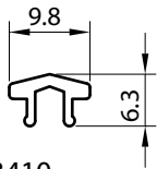
3410 GUIA INFERIOR Peso : 0.070 Kg/M Espesor : 1.3 mm Largo : 4.65 Mt.
