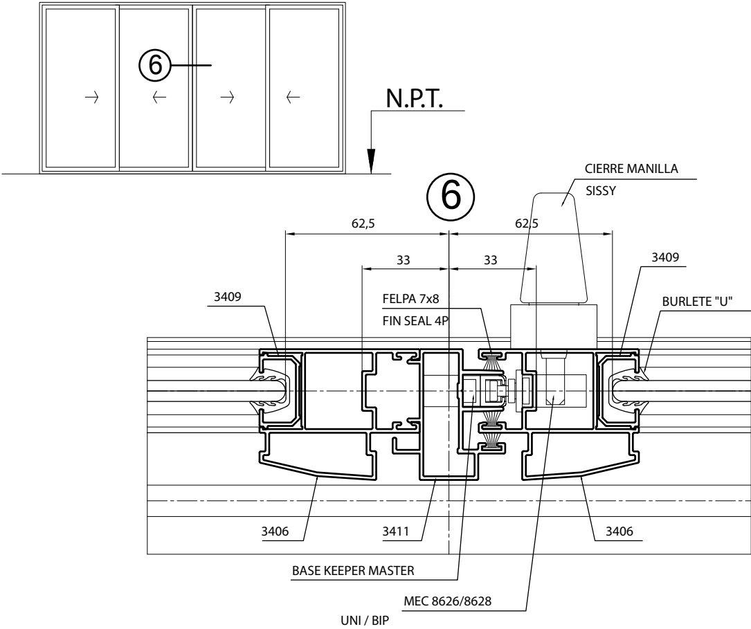
Corte Horizontal vidrio monolitico, encuentro a tope cuarta hoja.
